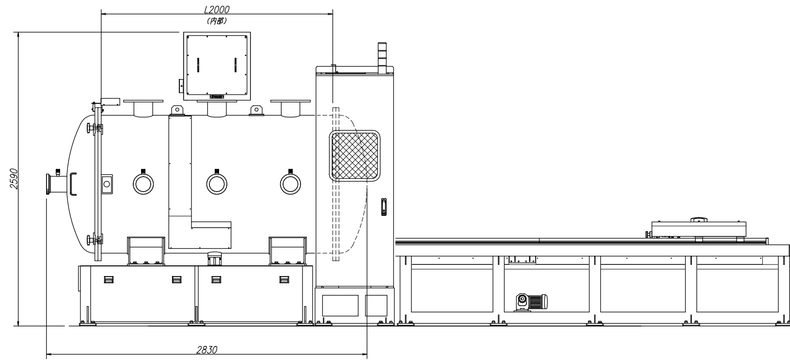
真空装置（正面）
