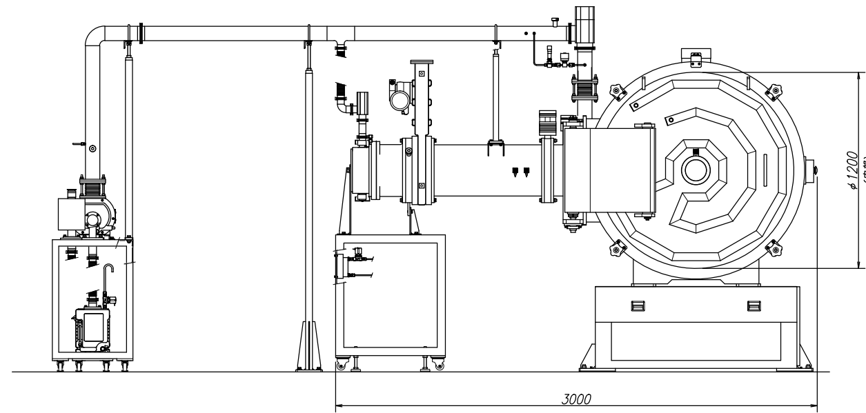
真空装置（左側面）
