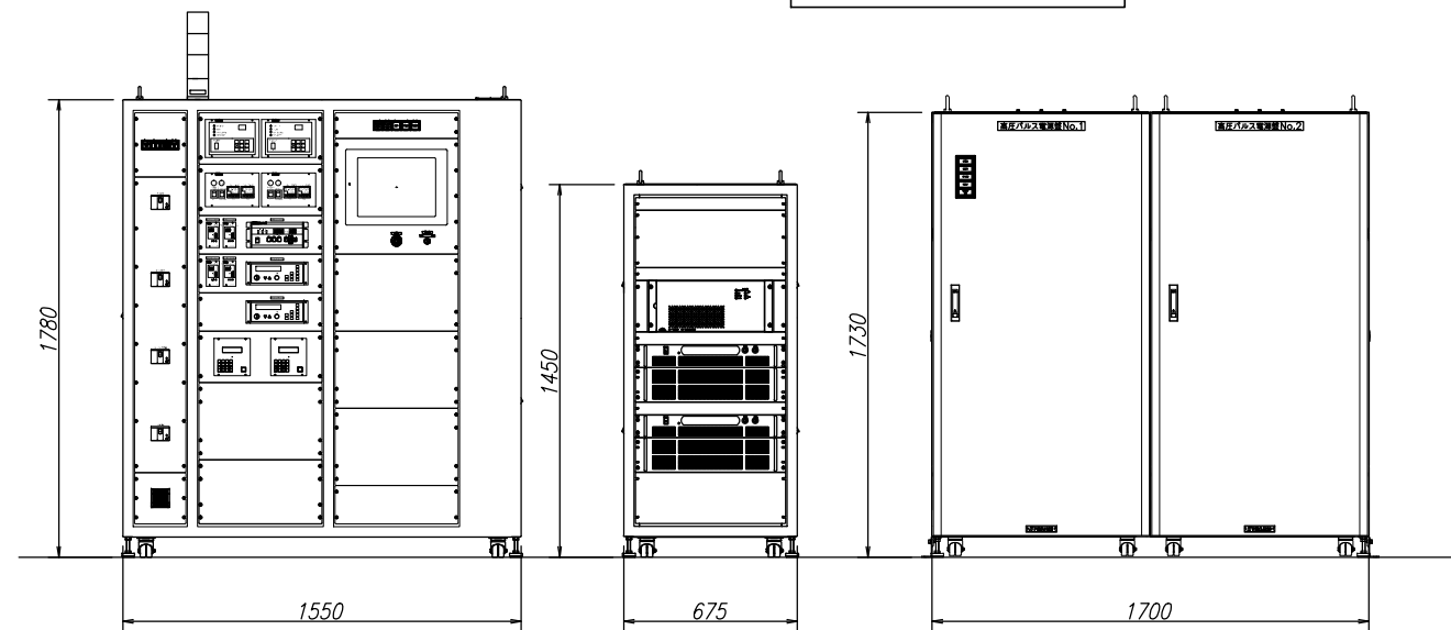
操作盤
